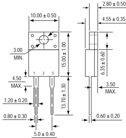
ITO-220AC
